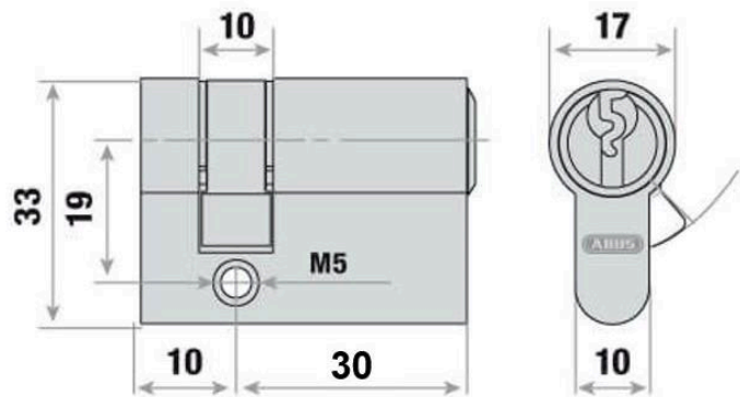
Artikel-Nr. 11916 Profilhalbzylinder für EURO 2000 + EURO 5000, 30/10 mm für Kühlraum-Drehtür Typ „KE“
