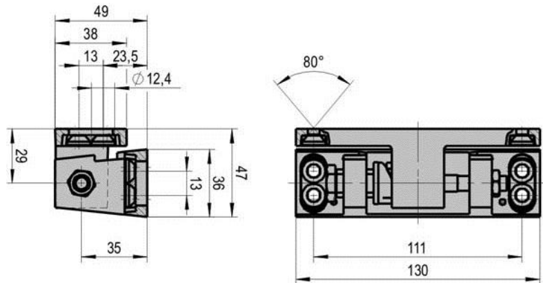
Artikel-Nr. 10203 Tiefkühlraumtür-Band, verchromt, DIN L Typ „Gastro 2“
