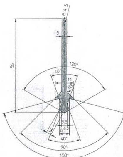
Artikel-Nr. 11122 Elastomerdichtung, schwarz für Pendeltür Typ „EPK“
