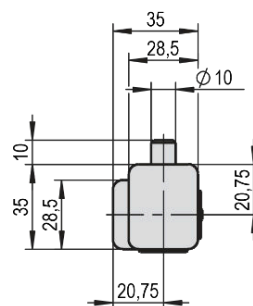
Artikel-Nr. 10204 3-tlg. VA-Band, steigend, höhenverstellbar für Betriebsraum-Drehtür Typ „EBF“
