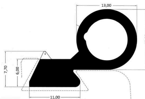
Artikel-Nr. 11007 Dichtungsgummi für Kühlraum-Drehtür Typ „Gastro KE/Gastro VE/Gastro 2 VE“
