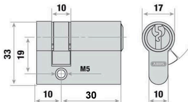
Artikel-Nr. 11916 Profilhalbzylinder für EURO 2000, 30/10 mm für Tiefkühlraum-Drehtür Typ „VE“
