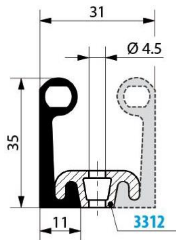
Artikel-Nr. 12000 Bodengummi für Schiebetüren Typ „LTS/LKS/LBS“
