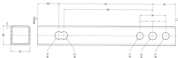
Artikel-Nr. 13783 Unterlage für 3-tlg. VA-Band steigend und nicht steigend für Tiefkühlraumtür-Band Typ „VE“
