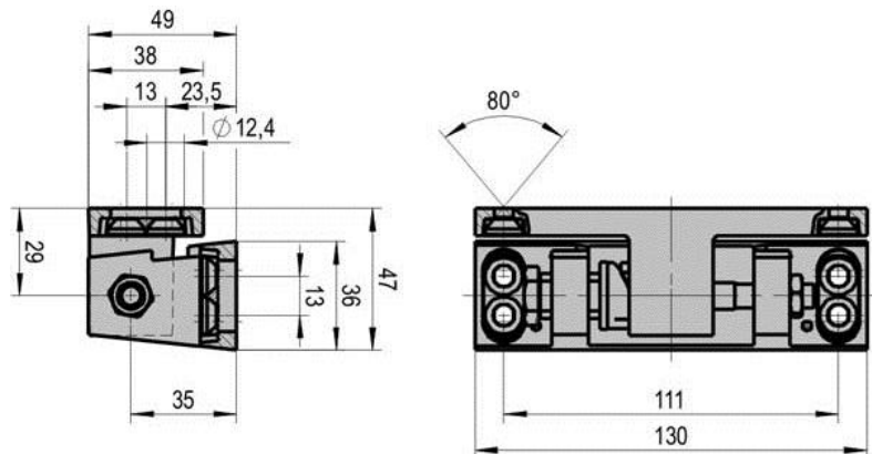
Artikel-Nr. 10202 Tiefkühlraumtür-Band, verchromt, DIN R Typ „Gastro 2“
