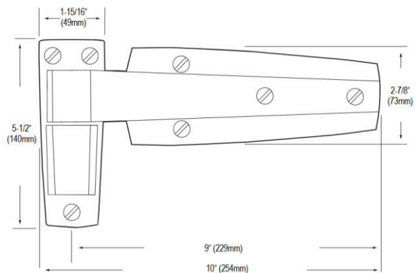
Artikel-Nr. 11118 Keilband verchromt, steigend mit Überschlage Typ „Gastro“
