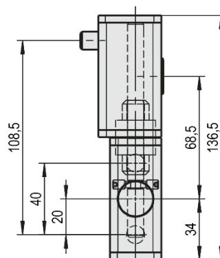
Artikel-Nr. 10204 3-tlg. VA-Band, steigend, höhenverstellbar für Betriebsraum-Drehtür Typ „EBF“
