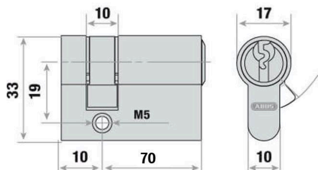
Artikel-Nr. 13792 Profilhalbzylinder, 70/10 mm für Langschild VA für Kühlraum-Drehtür Typ „KE“
