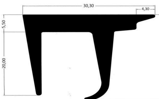
Artikel-Nr. 11005 Bodengummi mit Aluleiste für Kellertür Typ „KFE“
