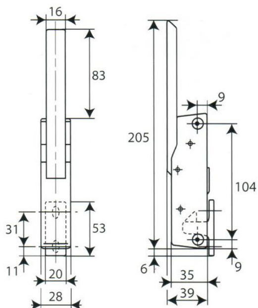
Artikel-Nr. 11113 Lukenschloss verchromt 880, nicht abschließbar für Kühlraum-Drehtür Typ „KE“
