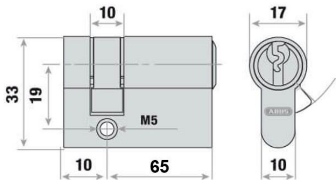
Artikel-Nr. 11648 Profilhalbzylinder, 65/10 mm für Langschild verchromt für Kühlraum-Drehtür Typ „KE“
