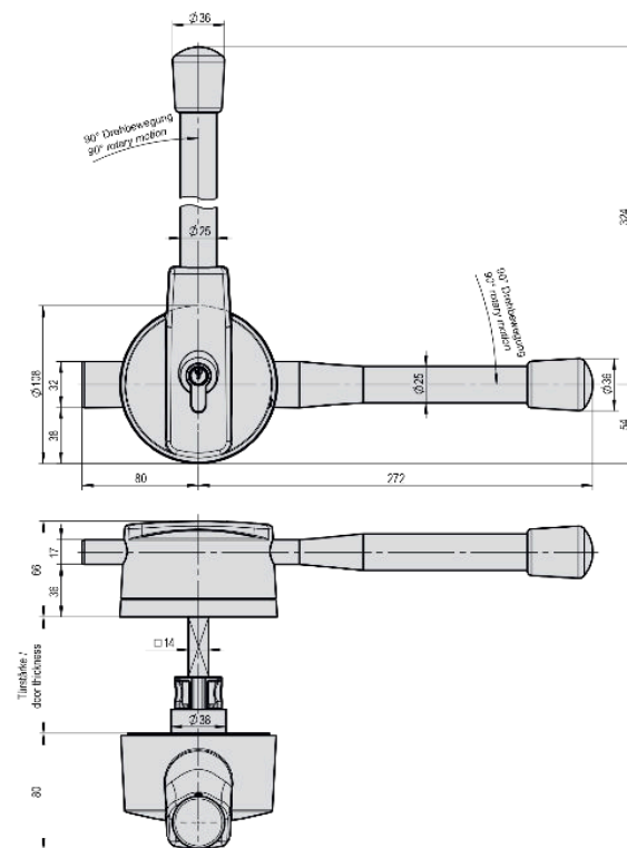
Artikel-Nr. 13701 EURO 5000 Presshebel für Tiefkühlraum-Drehtür Typ „VE“ für Türblatt-Stärke 140 mm
