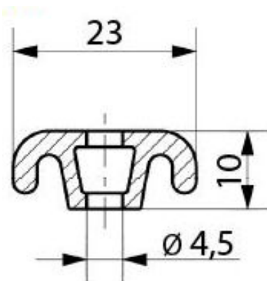
Artikel-Nr. 11734 Befestigungsleiste für Bodengummi Typ „LTS/LKS/LBS“
