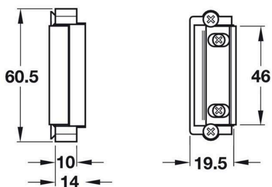
Artikel-Nr. 11123 Fafix Austauschstück für Betriebsraum-Drehtür Typ „EBF“
