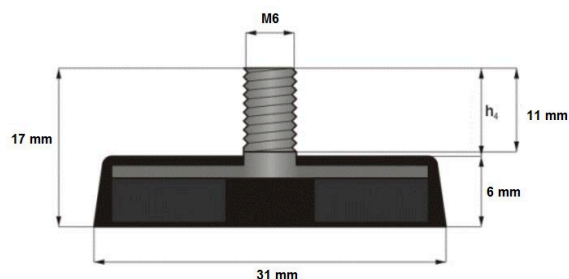
Artikel-Nr. 13764 Haftmagnet DM 31,0 x 6,0 mm gummiert Typ „Gastro 2“
