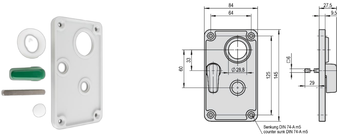
Artikel-Nr. 10958 Kunststoff Innenschild mit Notauslösevorrichtung für Tiefkühlraum-Drehtür Typ „VE“
