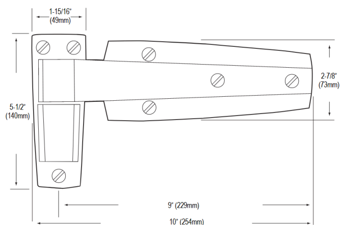
Artikel-Nr. 11117 Keilband verchromt, steigend ohne Überschlag Typ „Gastro“
