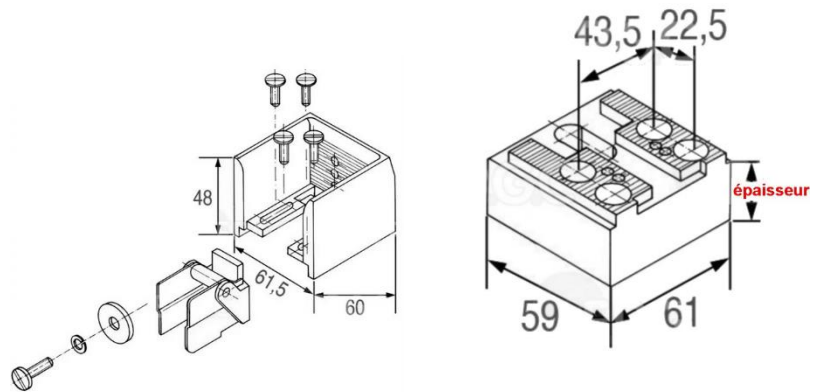
Artikel-Nr. 11793-1 Schließkloben für 30-43 mm Türblatt-Überschlag für Kühlraum-Drehtür Typ „KE“
