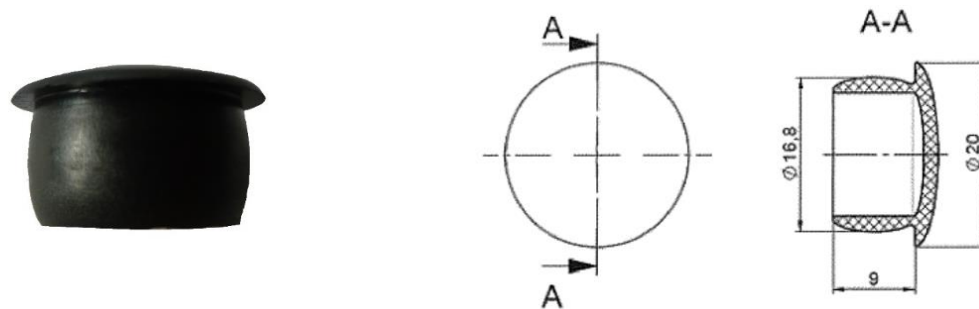
Artikel-Nr. 13725 Abdeckkappe rund für 3-tlg. Band Typ „EBF“, neue Version
