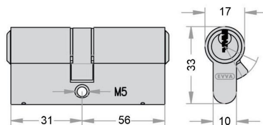
Artikel-Nr. 11870 Profildoppelzylinder 31/56 mm für Kellertür Typ „KFE“
