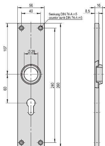
Artikel-Nr. 13665 Langschild verchromt, inkl. Kunststoffring für Tiefkühlraum-Drehtür Typ „VE“ (Auslaufmodell; zeitlich begrenzt lieferbar)
