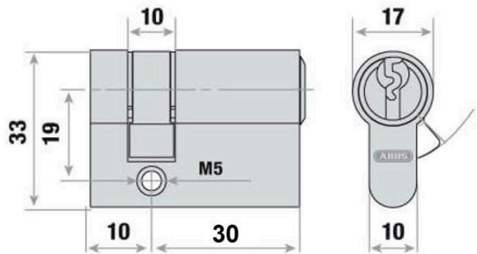
Artikel-Nr. 11916 Profilhalbzylinder 30/10 mm für EURO 2000 + EURO 5000, für Kühlraum-Drehtür Typ „KE“
