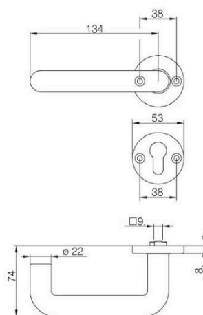
Artikel-Nr. 10111-1 Drückergarnitur in Edelstahl mit Rundrosette für Kellertür Typ „KFE“
