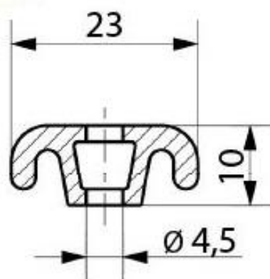
Befestigungsleiste für Bodengummi Typ „LTS/LKS/LBS“
