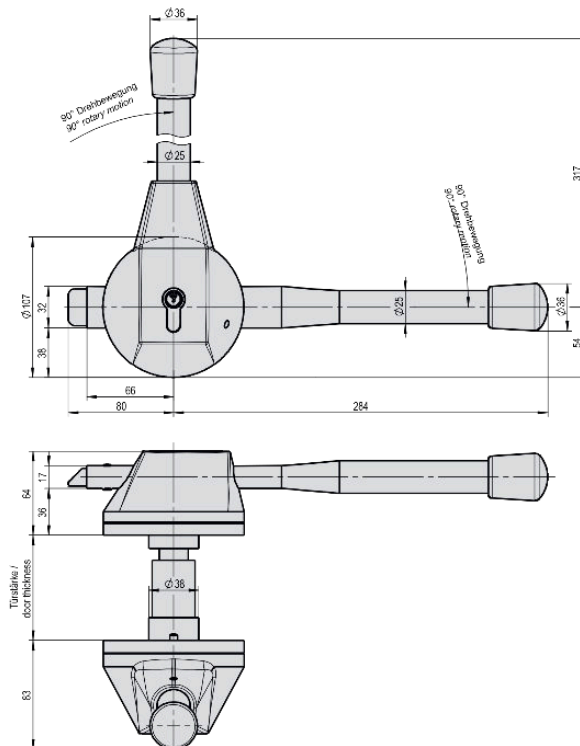
Artikel-Nr. 10179 EURO 2000 Presshebel für Tiefkühlraum-Drehtür Typ „VE“ für Türblatt-Stärke 136-140 mm
