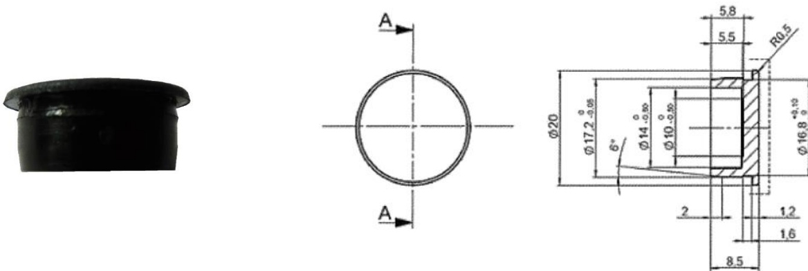
Artikel-Nr. 11683 Abdeckkappe rund für 3-tlg. Band Typ „EBF“, alte Version
