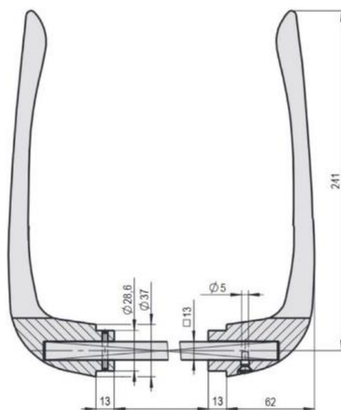
Artikel-Nr. 10211 Presshebel verchromt für Kühlraum-Drehtür Typ "KE" für Türblatt-Stärke 82-90 mm
