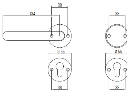
Artikel-Nr. 10110-1 Knopf-Drückergarnitur in Edelstahl mit Rundrosette für Kellertür Typ „KFE“
