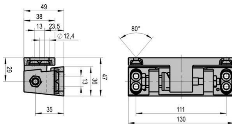
Artikel-Nr. 10203 Tiefkühlraumtür-Band, steigend, verchromt, DIN L Typ „VE“
