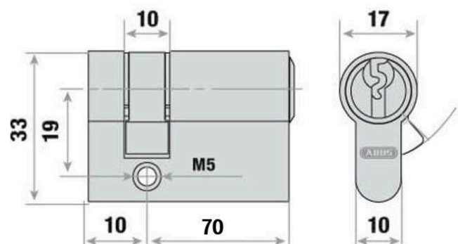
Artikel-Nr. 13792 Profilhalbzylinder, 70/10 mm für Langschild VA für Kühlraum-Drehtür Typ „KE“
