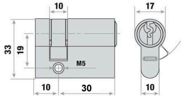
Artikel-Nr. 11916 Profilhalbzylinder 30/10 mm für EURO 2000 + EURO 5000 für Tiefkühlraum-Drehtür Typ „VE“
