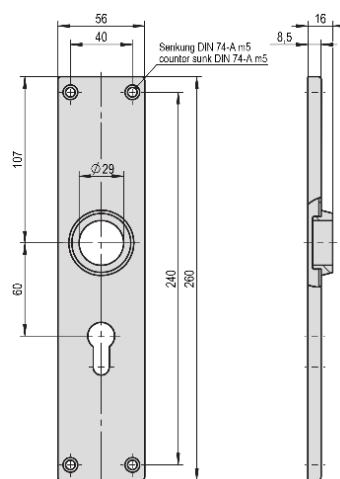
Artikel-Nr. 13665 Langschild verchromt, inkl. Kunststoffring für Kühlraum-Drehtür Typ „KE“ (Auslaufmodell; zeitlich begrenzt lieferbar)
